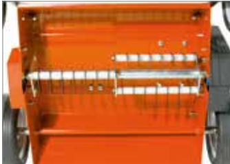
Rotore con 28 coltelli flottanti montati su cuscinetti a sfera e sistema di ingrassatore.
